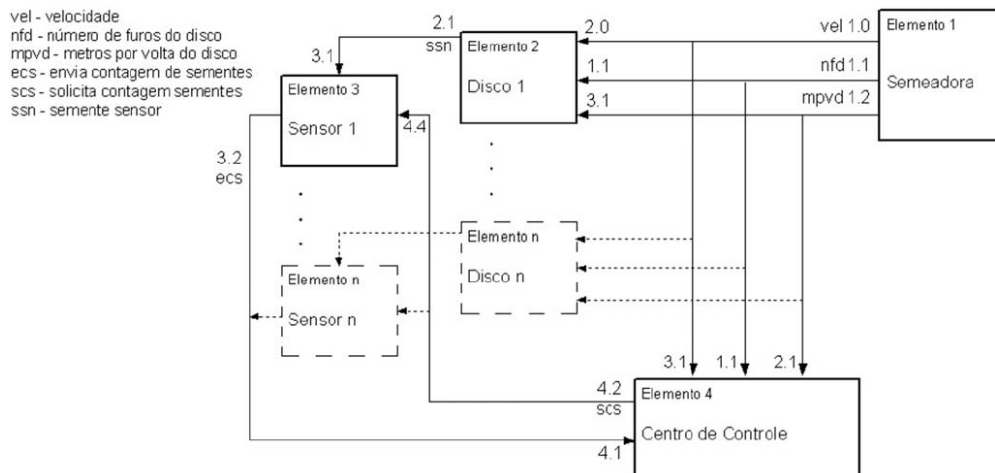
Figura 4. Arquitetura do SEP.
