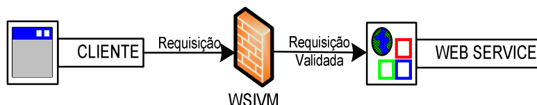
Figura 5. Requisição SOAP com WSIVM.
