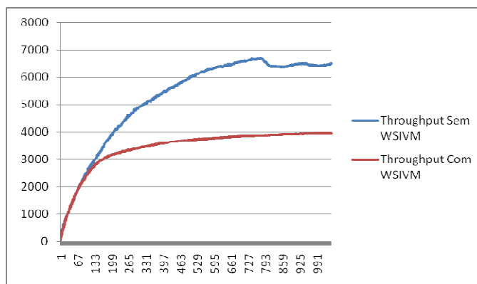
Figura 14. Throughput com e sem validação WSIVM.
