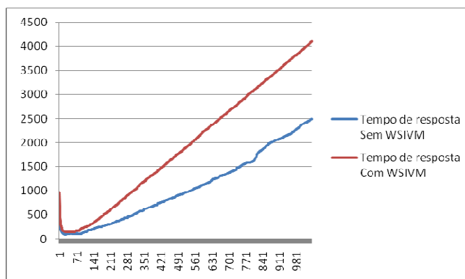
Figura 13. Tempos de resposta com e sem o uso do WSIVM.
