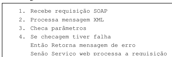
Figura 7. Algoritmo da Validação das Mensagens.
