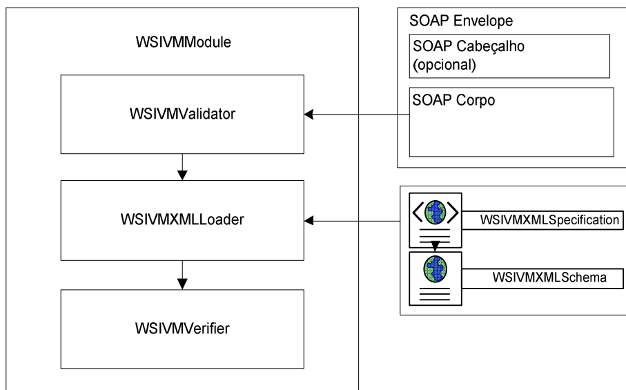
Figura 8. Funcionamento do WSIVM.
